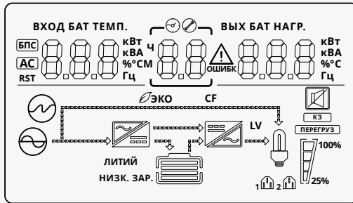
Рис. 17 LCD-дисплей
